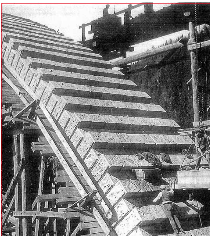
Rys. 5. Układanie kłińców kamiennych sklepienia mostu przez Prut pod Jaremczem
