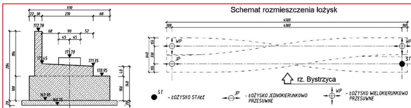
Rys. 9. Łożyska mostu: a) ciös podłożyskowy; b) łożyskowanie
