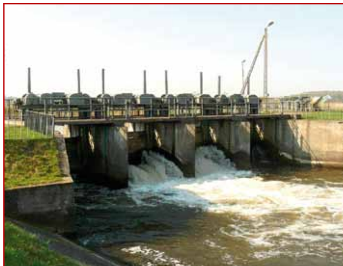
Ujęcie wody z rzeki Wieprz do Kanału Wieprz-Krzna
