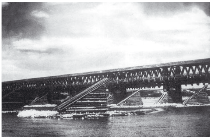
Rys. 3. Most drewniany kratownicowy przez Wisłę w Annopolu o dł. 852 m. Rok 1916. Arch.
